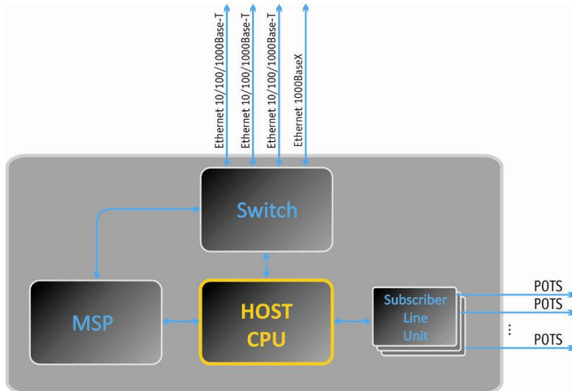
Рисунок 3б – Функциональная схема TAU-36.IP
