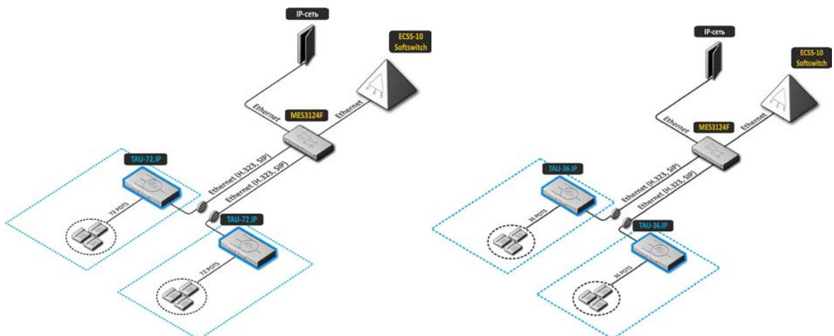
Рисунок 2 – Распределенная мини АТС TAU-72.IP/TAU-36.IP
